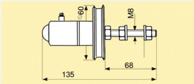
Рис. 2. Индикатор УЗА-220В. Габаритный чертёж
