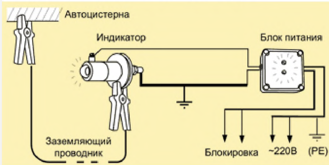
Рис. 4. Схема соединений
