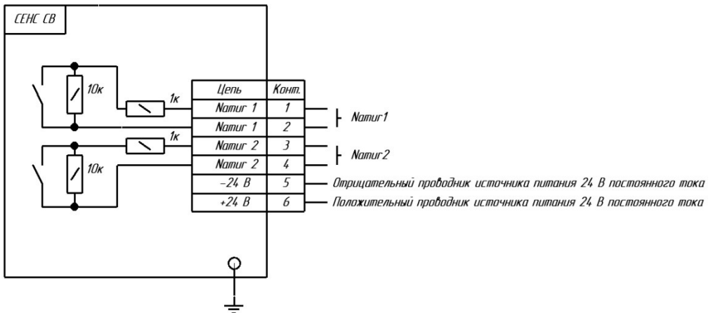
Рисунок Ж.2. Электрическое подключение сигнализатора. Выходной сигнал – Намур.
