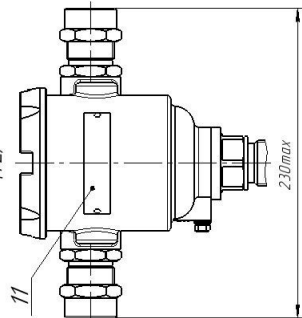
Рис. 3 Вариант с двумя кабельными вводами
